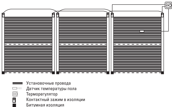
Рисунок 1. Общая схема подключения, в случаях, когда установочные провода проложены под плинтусом, утоплены в прорезях теплоизоляции, или в специальных кабель-каналах, исключая непосредственное механическое воздействие.
