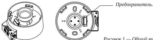
Рисунок 1 — Общий вид светильника СА-18
