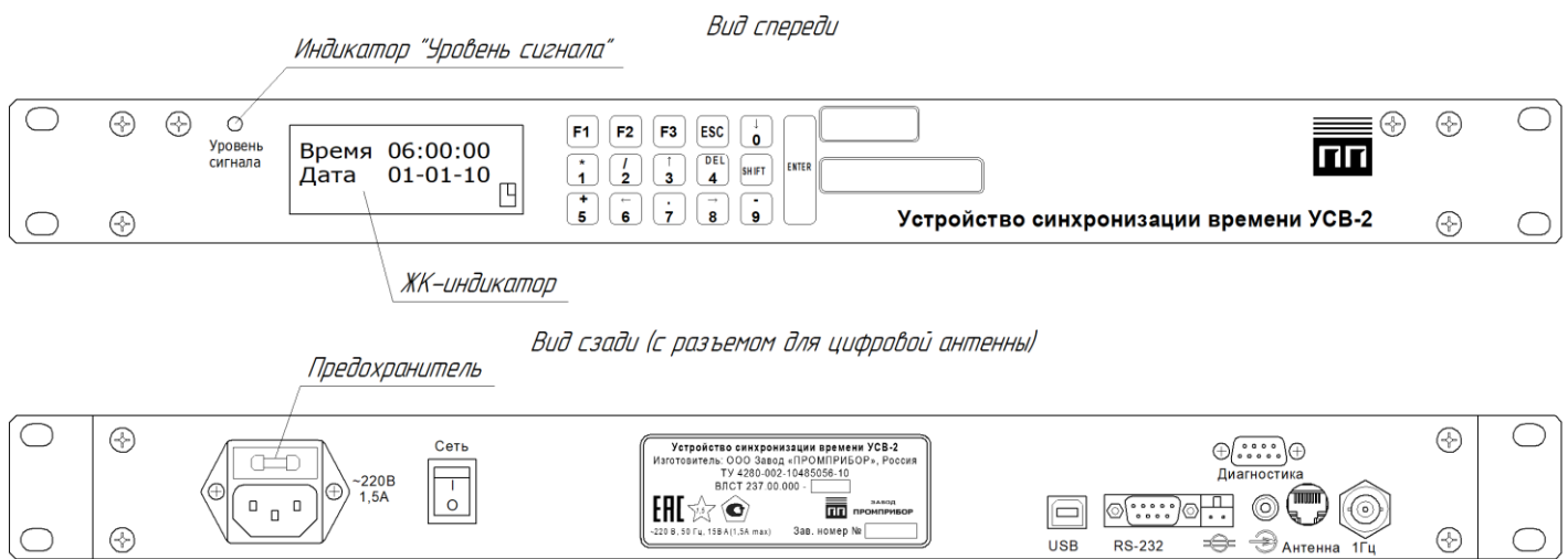
Рисунок 2.1 – Общий вид УСВ-2 ВЛСТ 237.00.000
