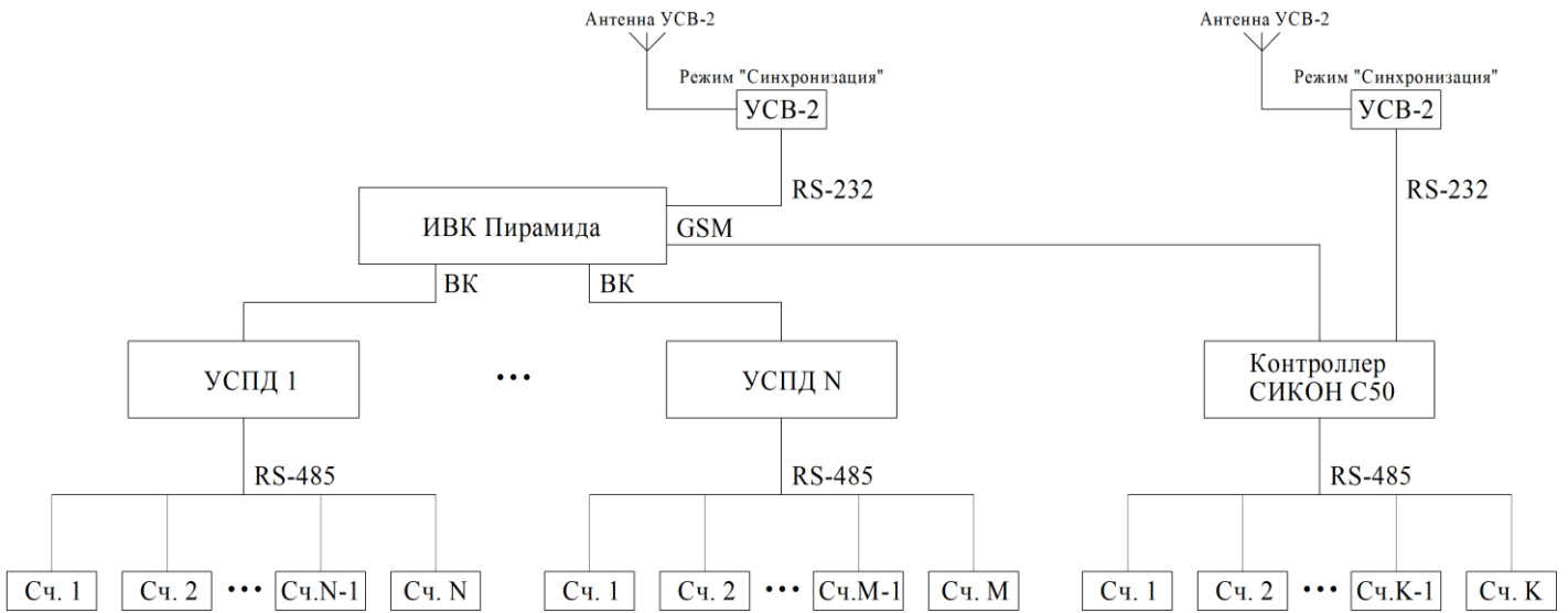
Рисунок В.1 – Типовая структурная схема СОЕВ УСВ-2
