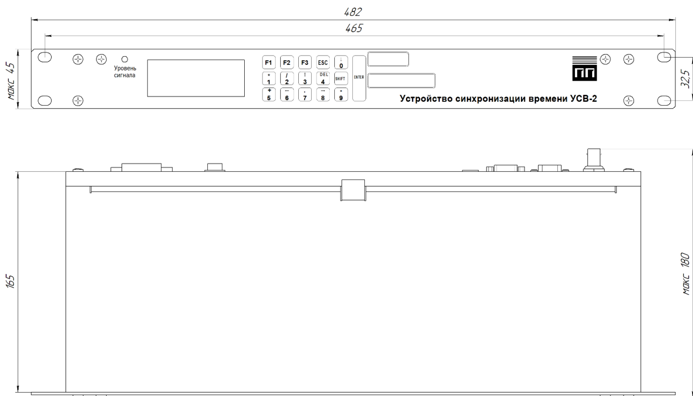
Рисунок Б.1 – Габаритные и установочные размеры УСВ-2 ВЛСТ 237.00.000
