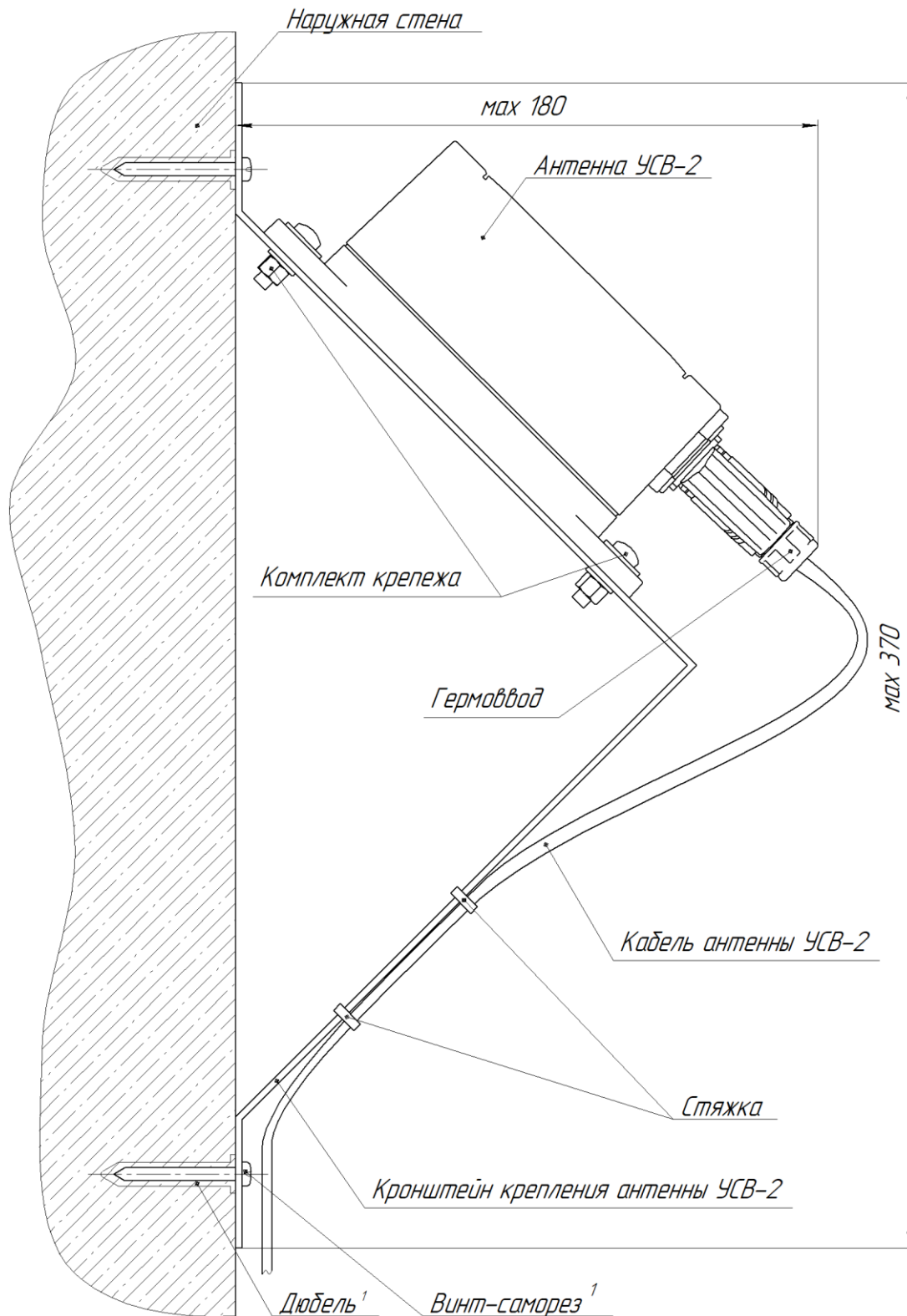
Рисунок Е.1 – Крепление антенны УСВ-2
